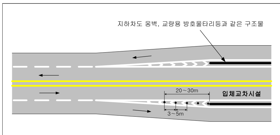
<그림 5.25> 입체교차를 위한 구조물 전방의 시선유도봉 설치 방법
