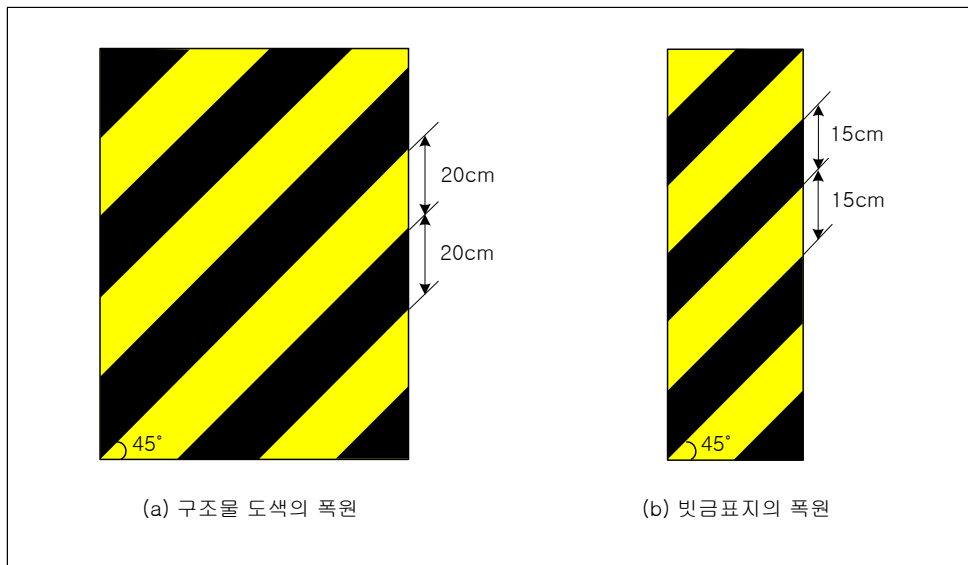
<그림 5.3> 구조물 도색 및 빗금표지의 폭원
